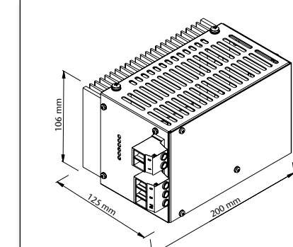
Optional DIN rail mount approx. 2.05 kg
