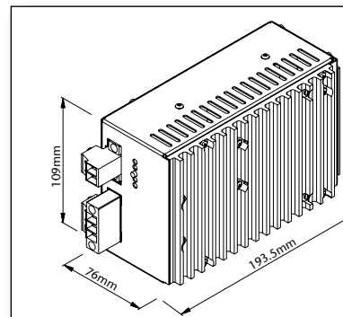
Optional DIN rail mount approx. 1.0 kg
